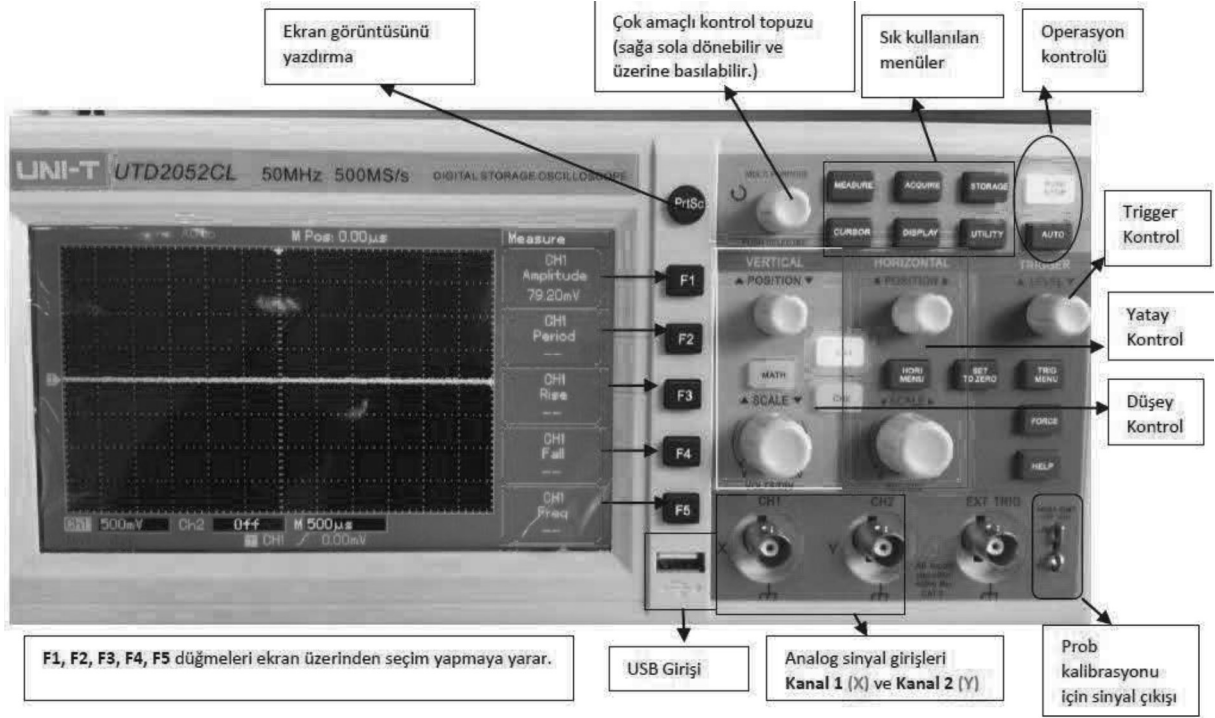
Şekil.13 Osiloskop Görünümü
