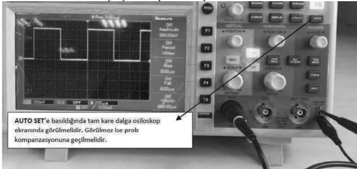
Şekil.17 Osiloskop görünümü
