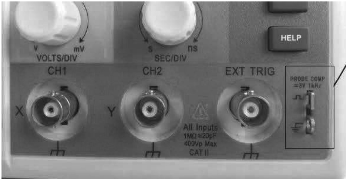
Şekil.16 Osiloskop Kalibrasyon Ekranı
