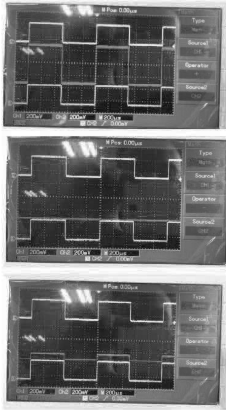
Şekil.27 Math fonksiyonu osiloskop çıktıları
