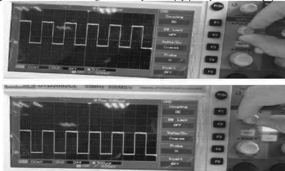
Şekil.21 Düsey ekran pozisyon kontrolü
