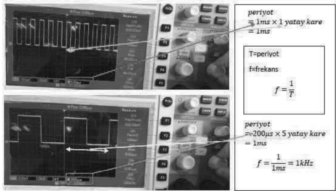
Şekil.24 Osiloskop yatay ölçkleme kontrolü
